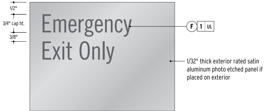
ALT DETAIL - EXTERIOR SCALE: 1" = 2"
