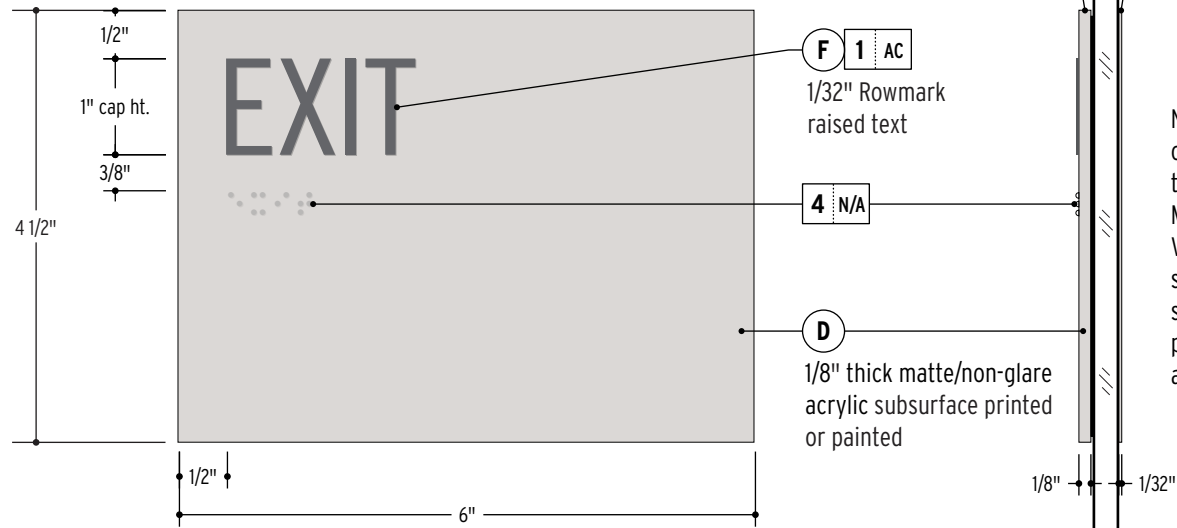
DETAIL SCALE: 1" = 2"
