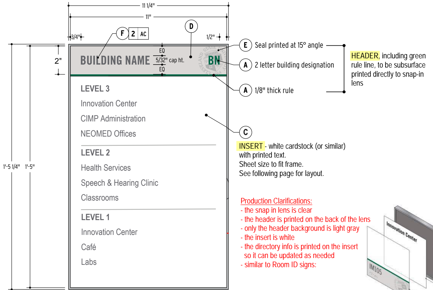
DETAIL SCALE: 3" = 1'
