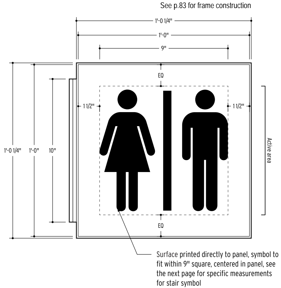
FRONT DETAIL SCALE: 3" = 1'-0"
