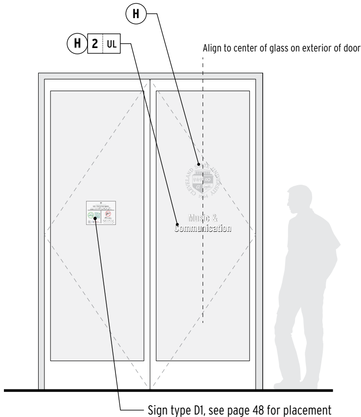
FRONT ELEVATION SCALE: 3/8" = 1'
