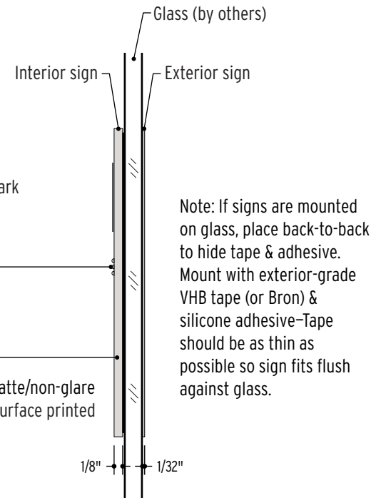
SECTION SCALE: 1" = 2"
