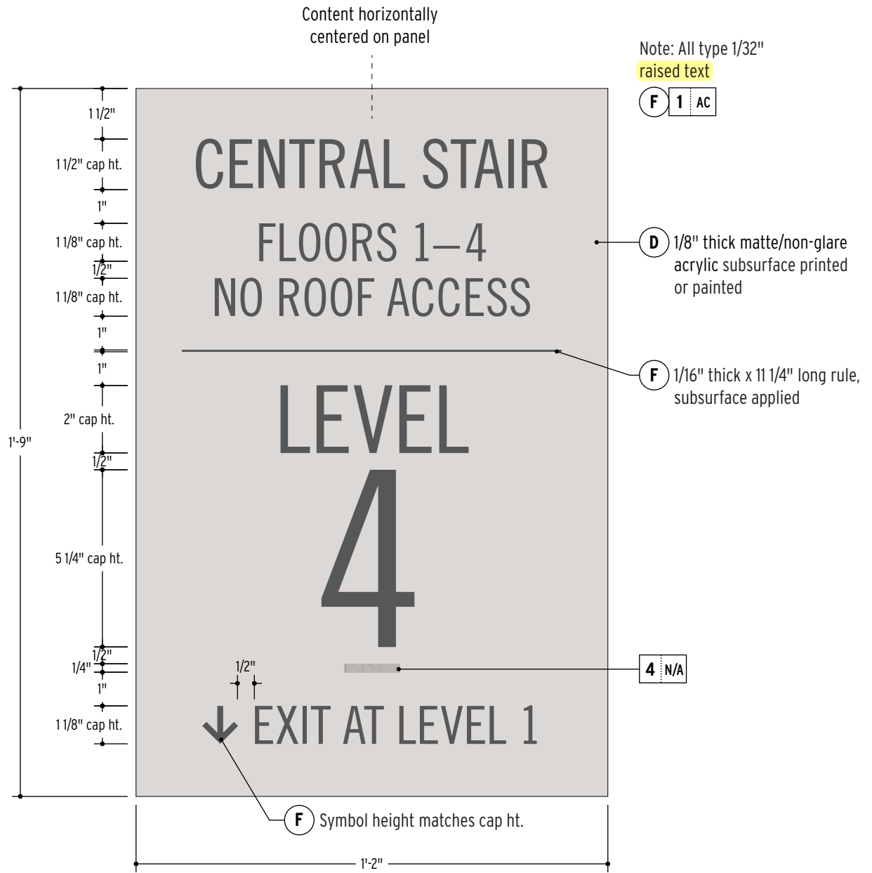
DETAIL SCALE: 3" = 1'
