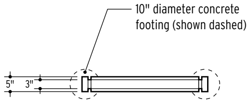
TOP SCALE: 3/8" = 1'-0"
