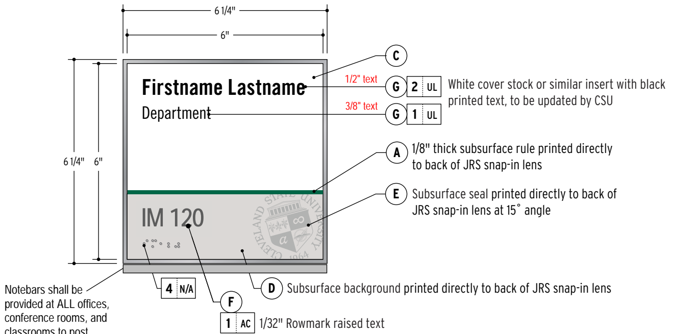
DETAIL SCALE: 1" = 3"
