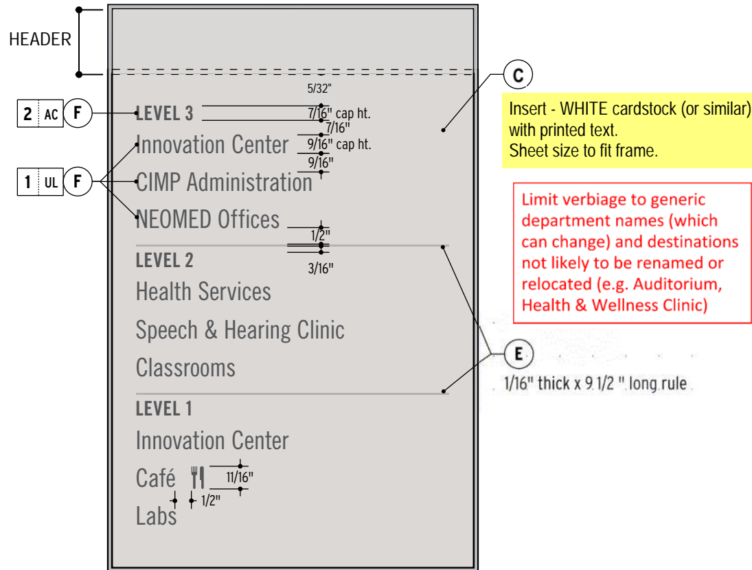
INSERT DETAIL SCALE: 3" = 1'
