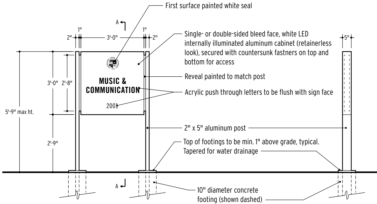
FRONT ELEVATION SCALE: 3/8" = 1'
