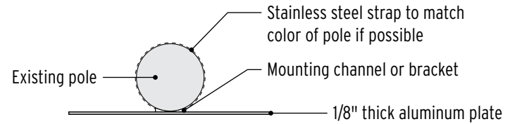
TOP SCALE: 1 1/2" = 1'
